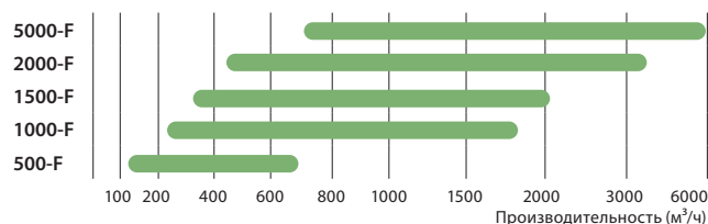
Типоразмеры и производительность ОТД-E
