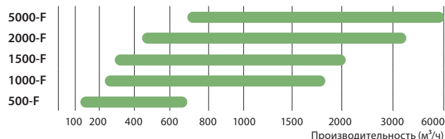
Типоразмеры и производительность ОТД-S
