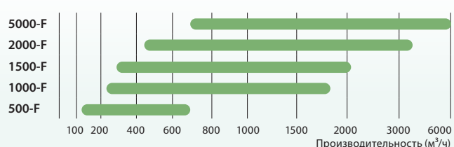
Типоразмеры и производительность ОТД-S
